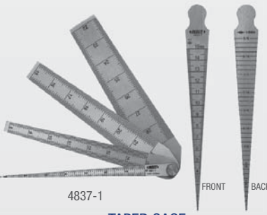
TAPER GAGE
